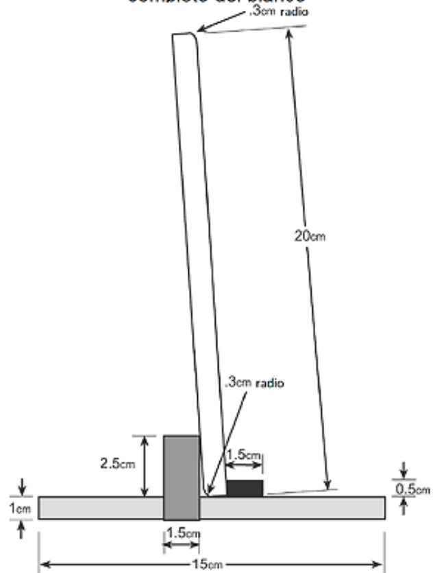
Alzado lateral completo del blanco
