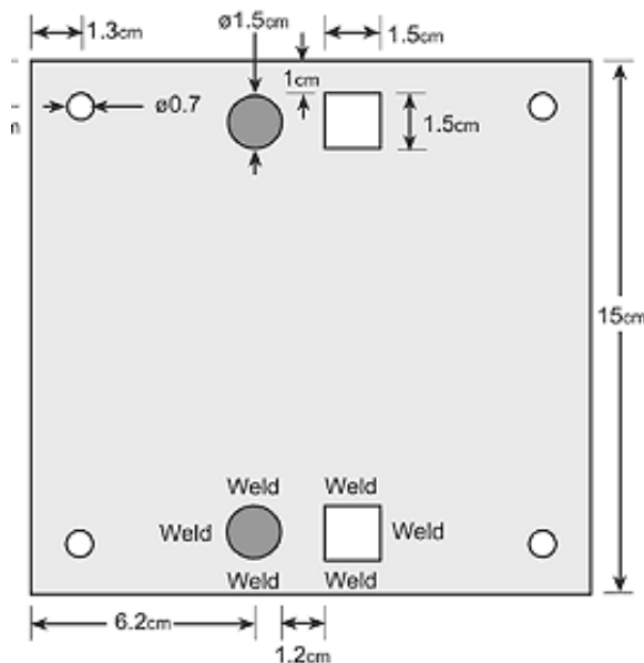
Base del blanco (vista de planta)
